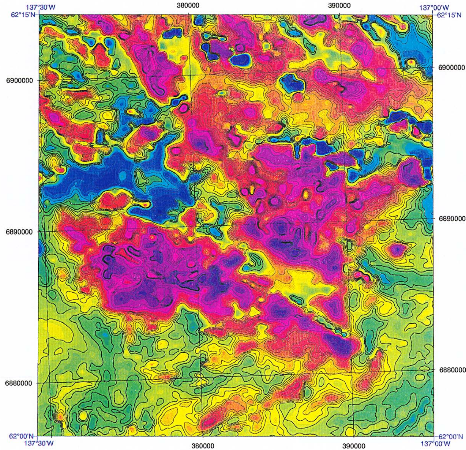
Residual Magnetic Total Field (nT) Champ total magnétique résiduel (nT)
