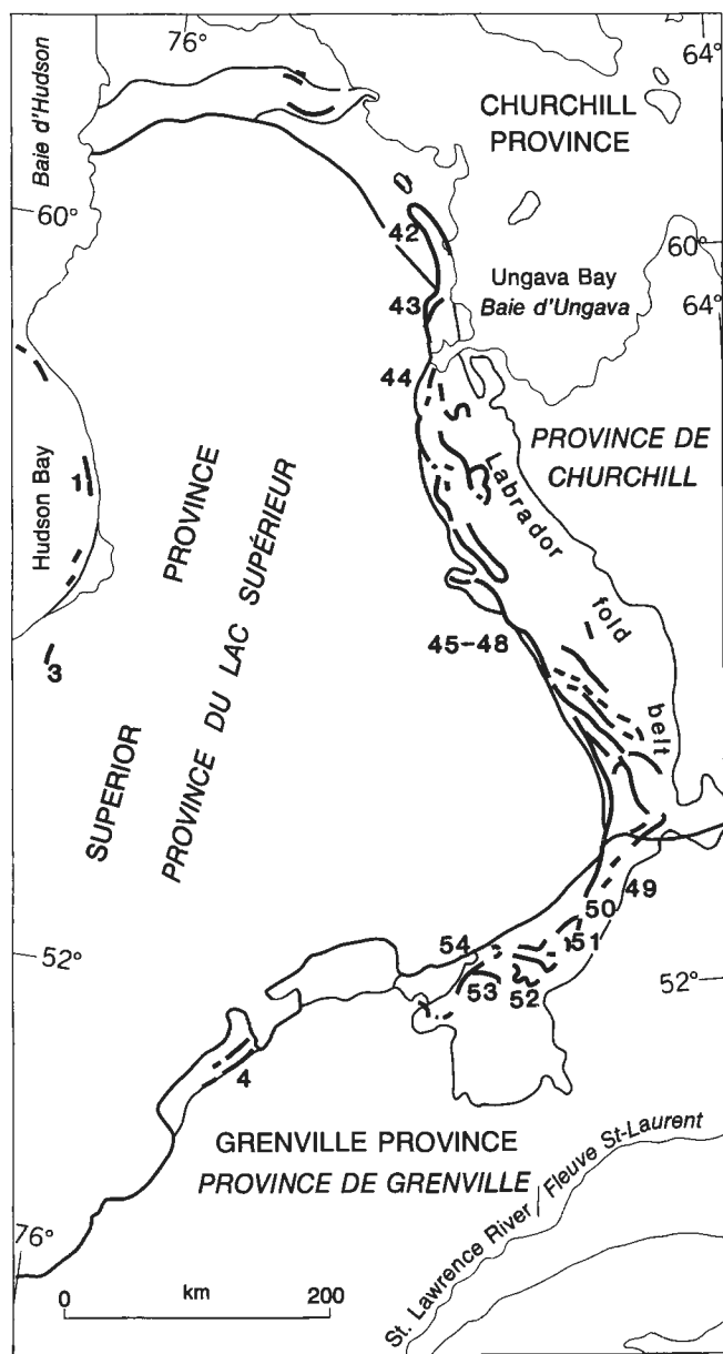
Figure 1B. Formations ferrifères au Québec et dans l'ouest du Labrador, Terre-Neuve. Les chiffres se rapportent aux formations identifiées au tableau 1.
