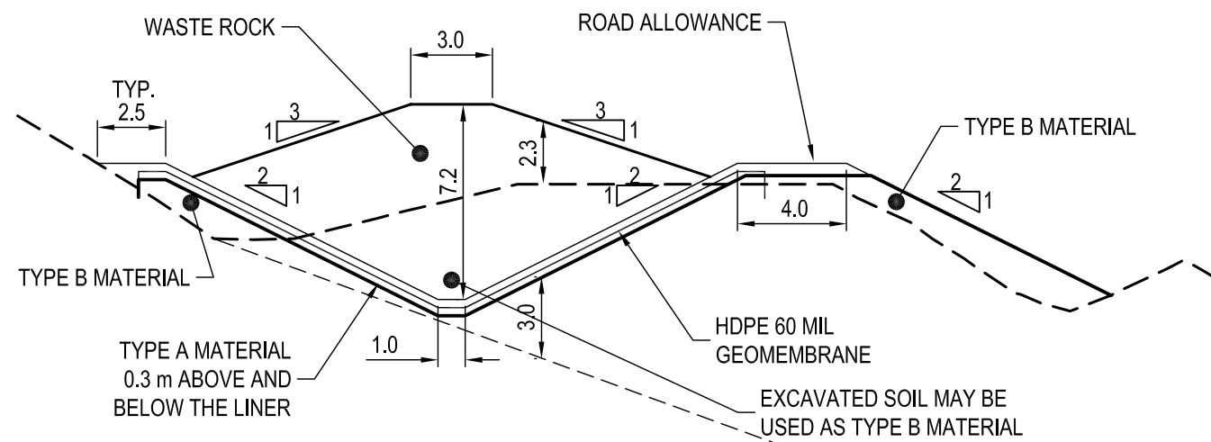
DETAIL 1 SCALE: 1 : 250 1
