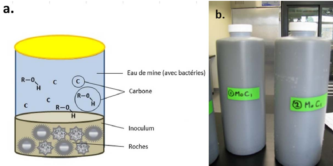
Figure 1-4 Bioreacteurs utilisés pour les essais en batch
