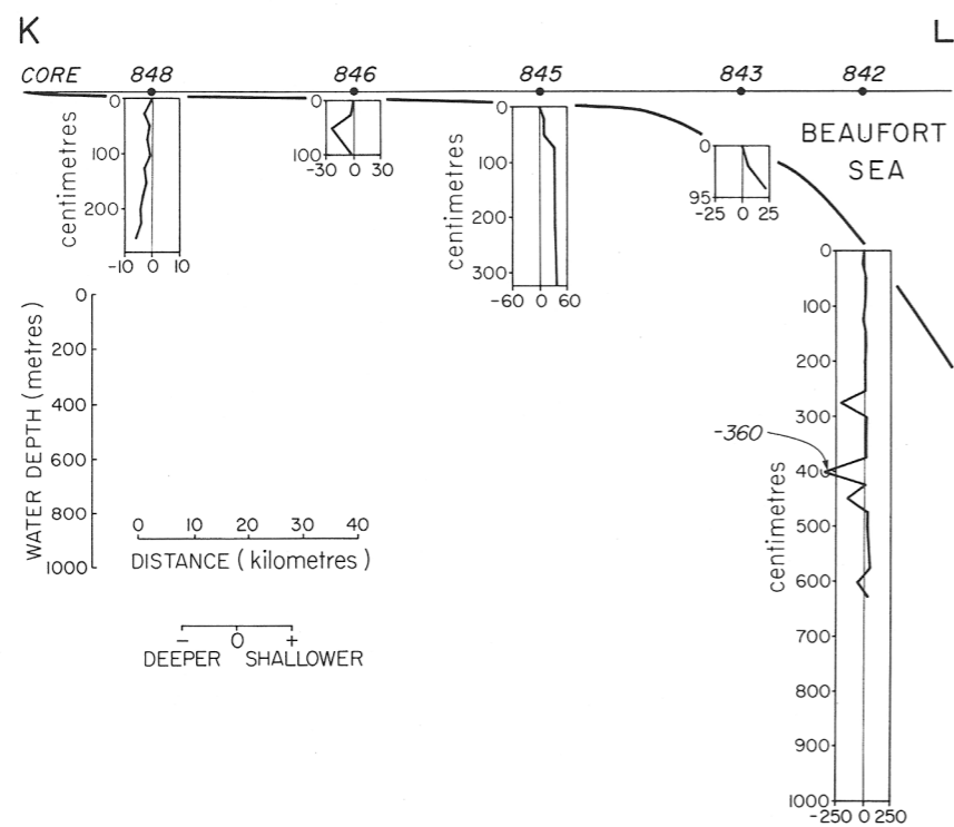
Figure 36. Traverse KL
